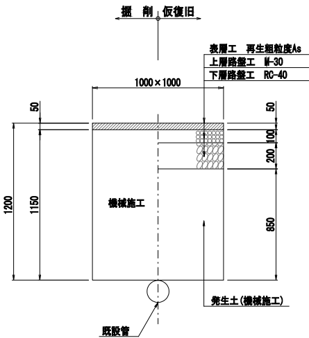
試掘箇所
