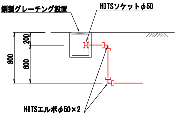
S - S 断面図 S=FREE
