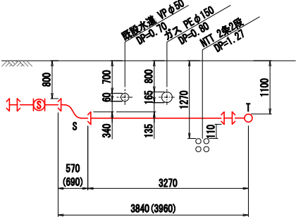
R - R 断面図 S=FREE
