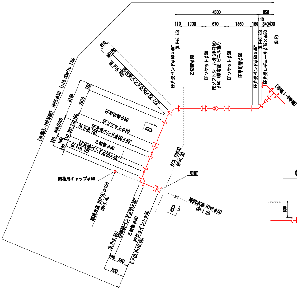
配管詳細図(1)参照 [市道 I-9号線]
