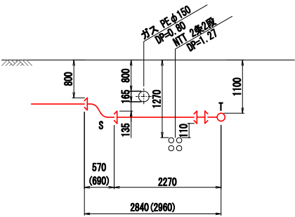
P - P 断面図 S=FREE
