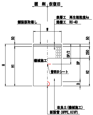
歩道 (布設)
