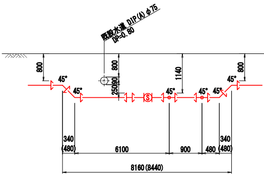
D - D 断面図 S=FREE
