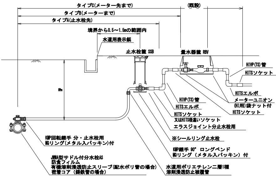
茨城県南水道企業団 標準配管図 タイプA,B,C (13mm～25mm)
