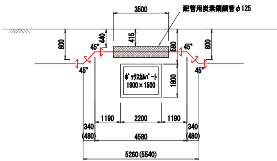
C - C 断面図 S=FREE
