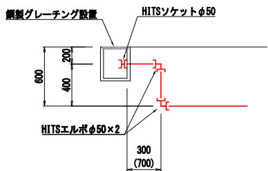
A' - A' 断面図 S=FREE
