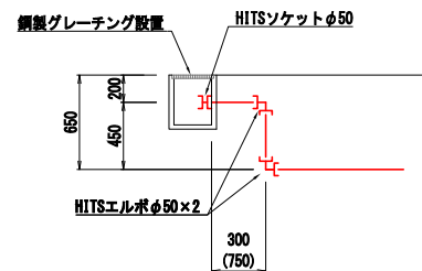
V - V 断面図 S=FREE
