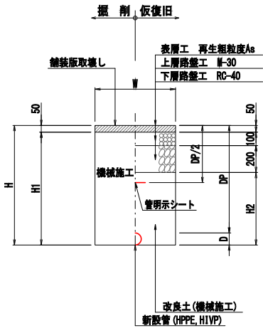
市道車道(B) (布設)
