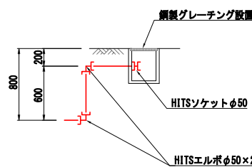
W - W 断面図 S=FREE
