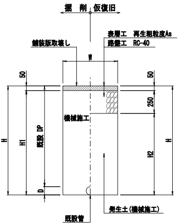
歩道 (撤去)
