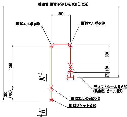
A' - A' 断面図 S=FREE
