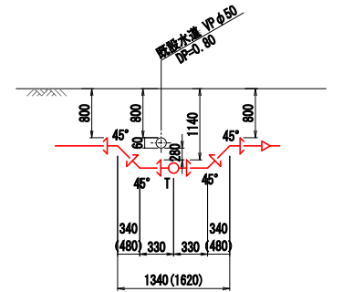
X - X 断面図 S=FREE
