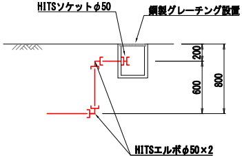
T - T 断面図 S=FREE
