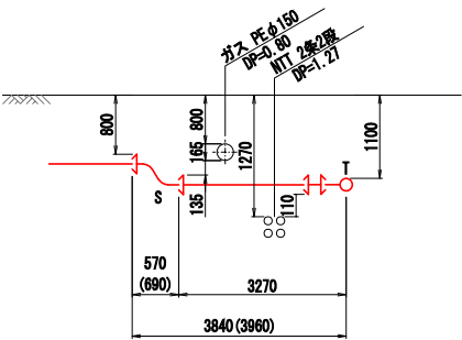
Q - Q 断面図 S=FREE
