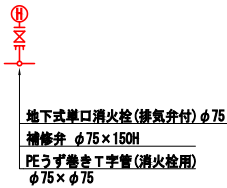
消火栓詳細図 S=FREE
