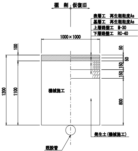
試掘箇所
