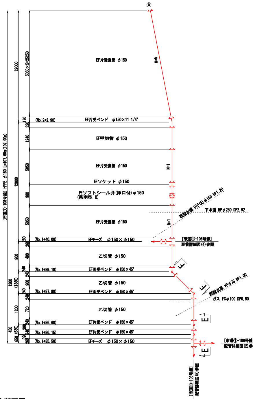
E - E 断面図 S=FREE
