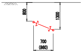
N - N 断面図 S=FREE
