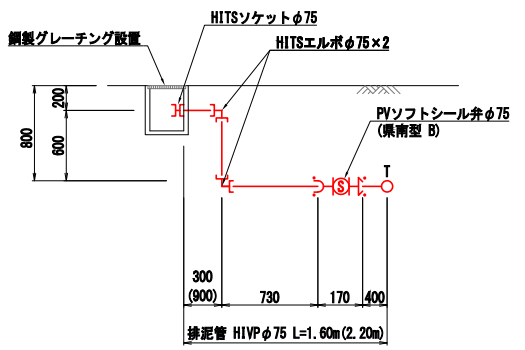
排泥管詳細図② S=FREE
