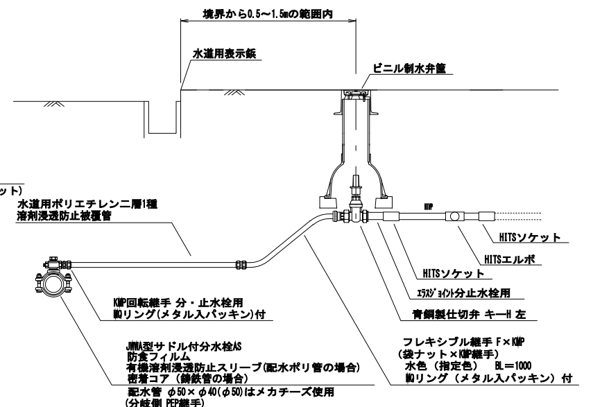
茨城県南水道企業団 標準配管図 タイプE (30mm~50mm)
