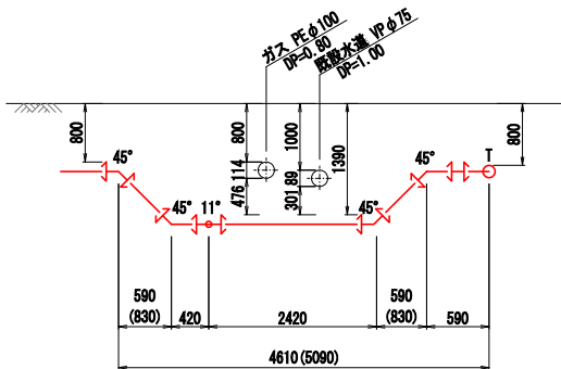
Q - Q 断面図 S=FREE
