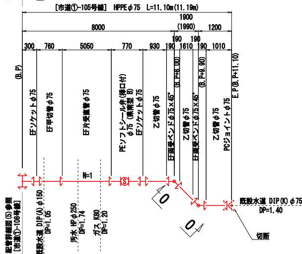
O - O 断面図 S=FREE
