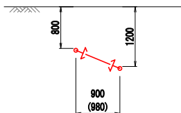
P - P 断面図 S=FREE
