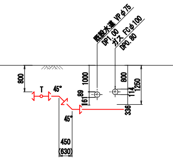
E - E 断面図 S=FREE
