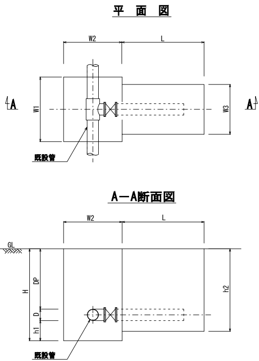
不断水割T字管土工図 S=Free (水平穿孔)
