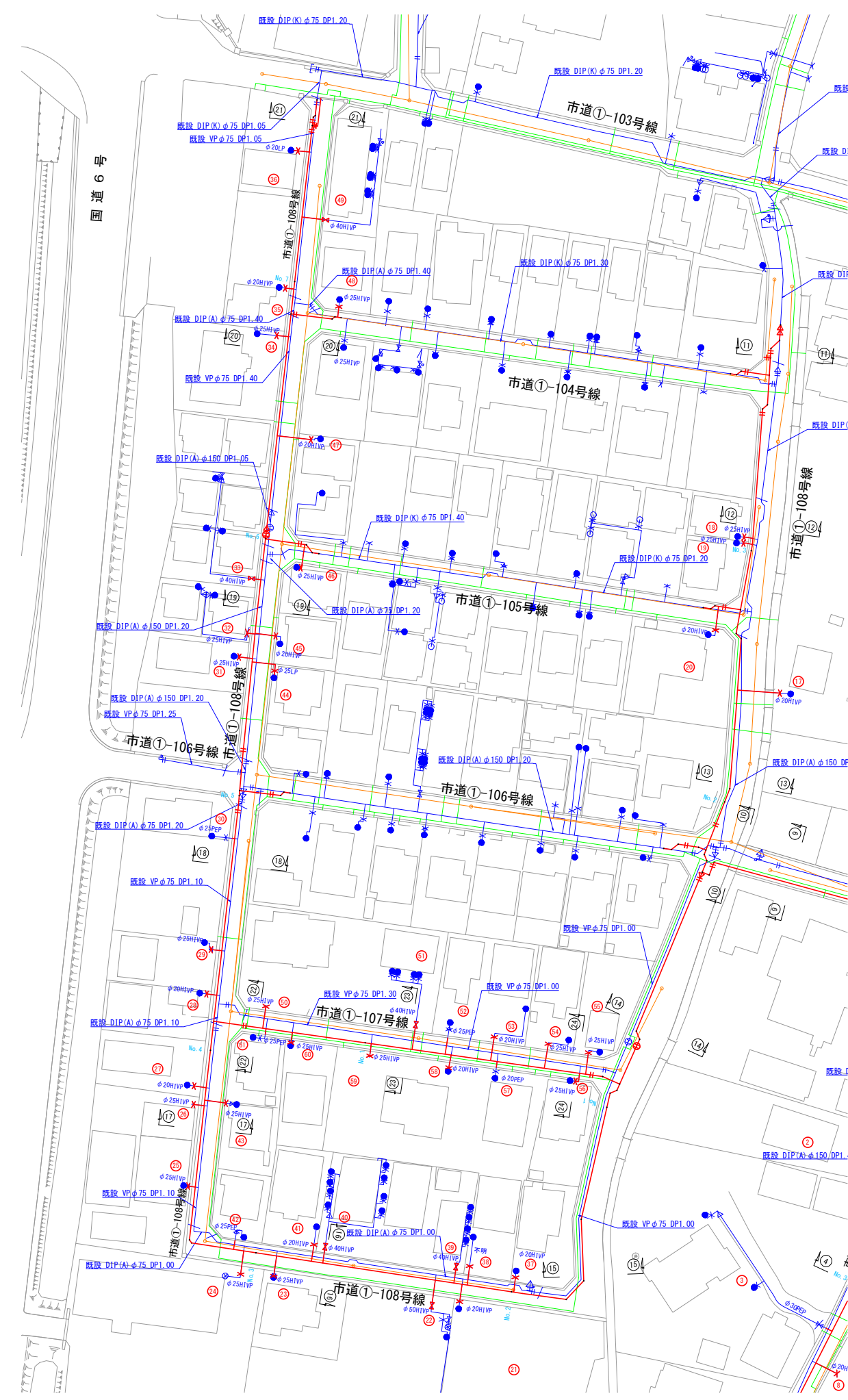
給水管平面図(3) S=1:500
