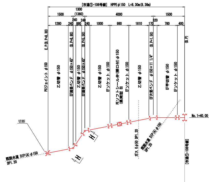
H - H 断面図 S=FREE
